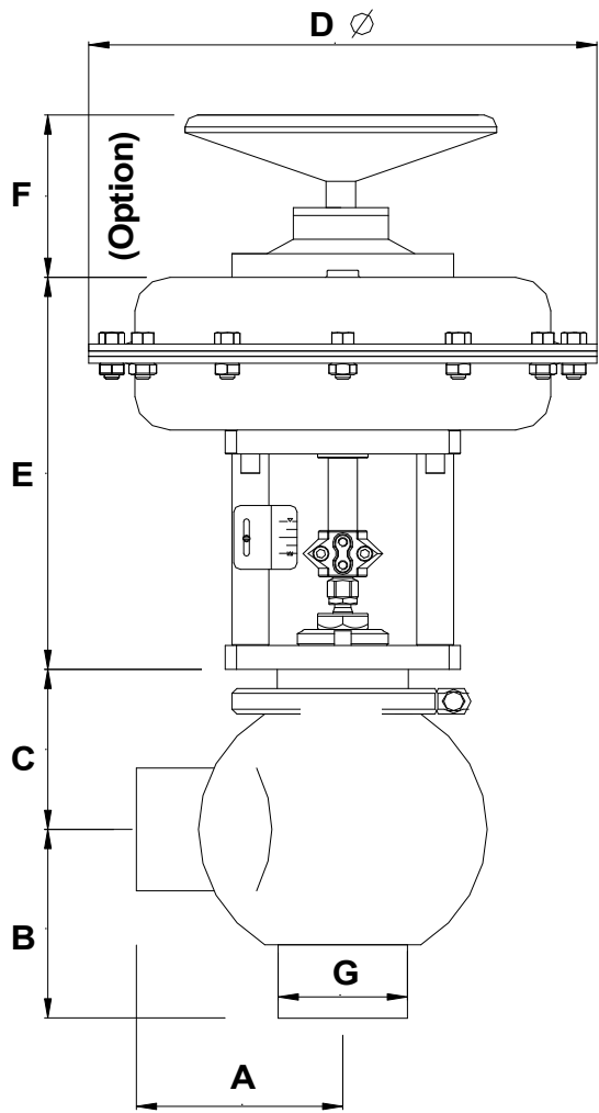
FLANGIA FLANGE
