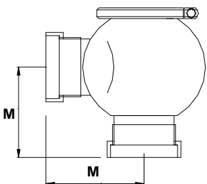
DIN FEMMINA DIN FEMALE
